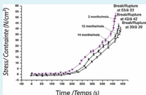
Figure 15 : Contrainte à la rupture pour une profondeur fixée à 4,4 mm à différentes durées de séjour en bouche. Rupture strain for a drilling depth fixed at 4.4 mm for different periods of stay in the mouth.
